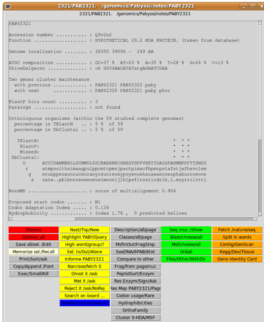
Figure 37 – Visualisation de l'annotation d'un PAB sous Gscope.
