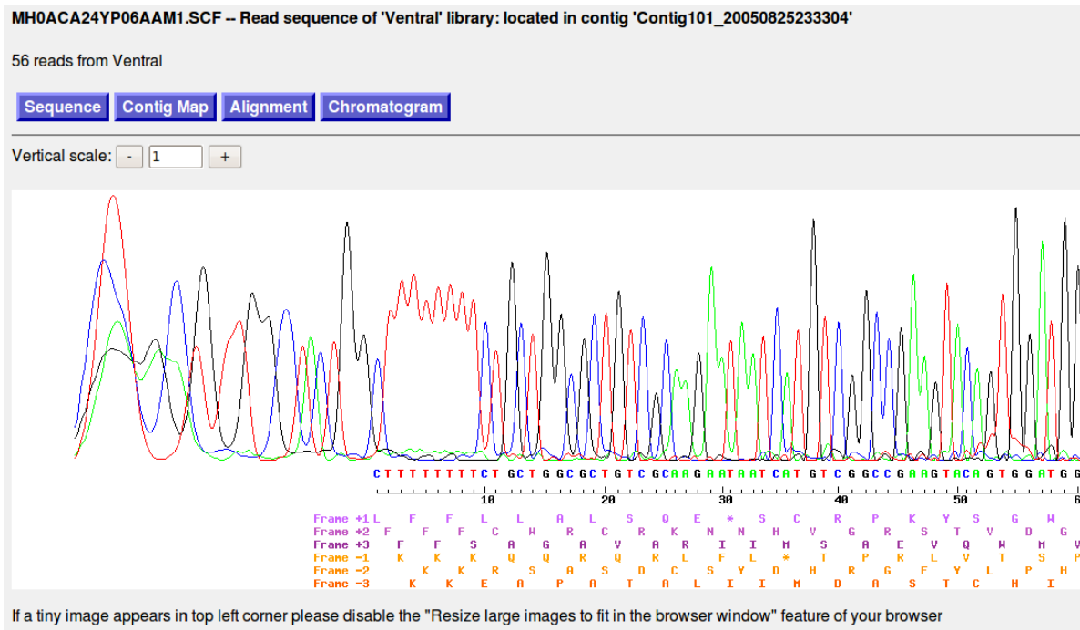
Figure 73 – Visualisation d'un chromatogramme
