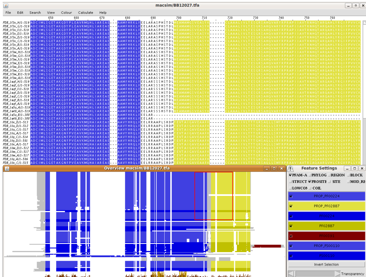
Figure 34 – Alignement multiple annoté par MACSIMS et visualisé dans Jalview
