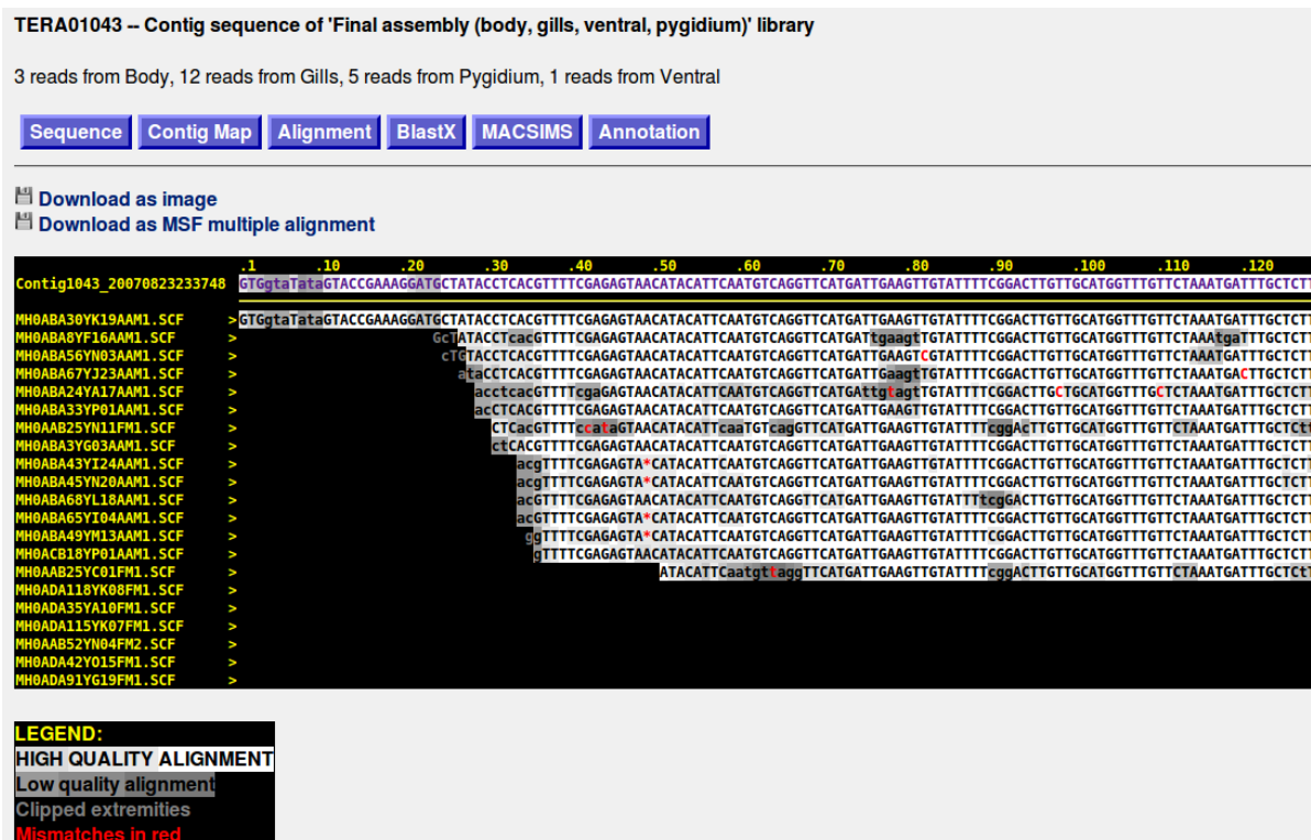
Figure 72 – Visualisation d'un contig sous forme d'alignement
