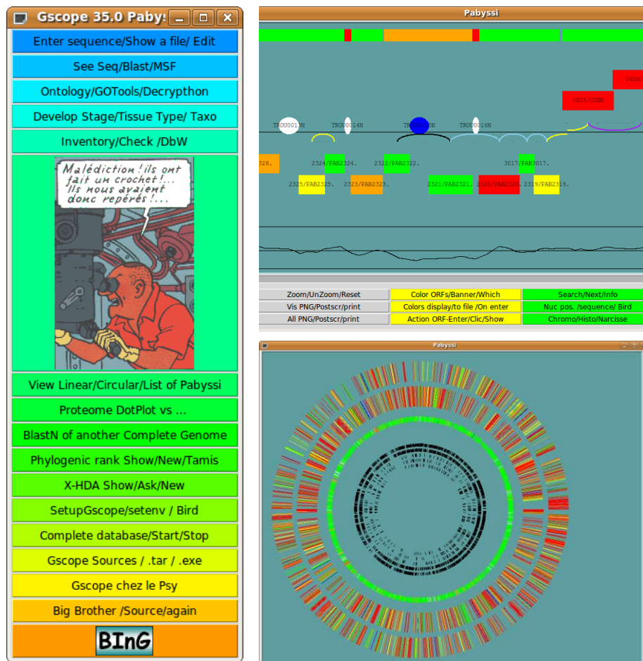
Figure 36 – Interface graphique de Gscope et aperçus du génome annoté de P.abyssi
