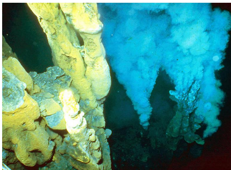
Figure 20 – Monts hydrothermaux laissant s'échapper des précipités métalliques
